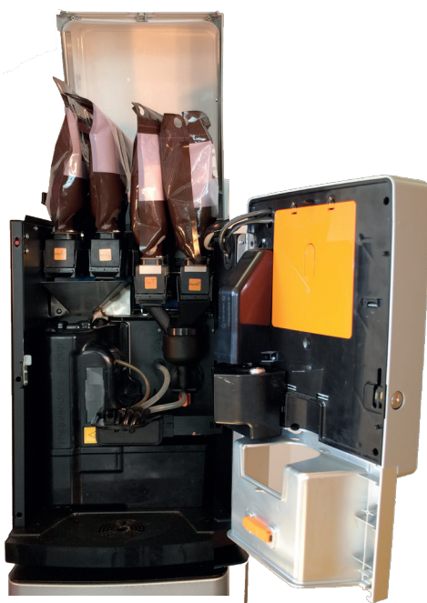
Intérieur du distributeur Cino eC café moulu avec le groupe et les 4 poches en place.
